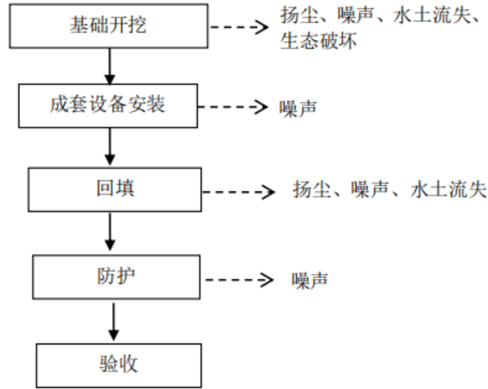
图 4-2 泵站修筑工艺流程及产污环节图
