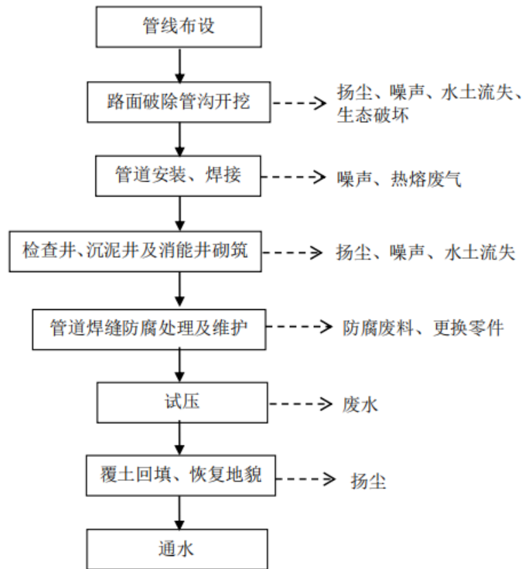
图 4-1 管网施工流程及产污环节图
