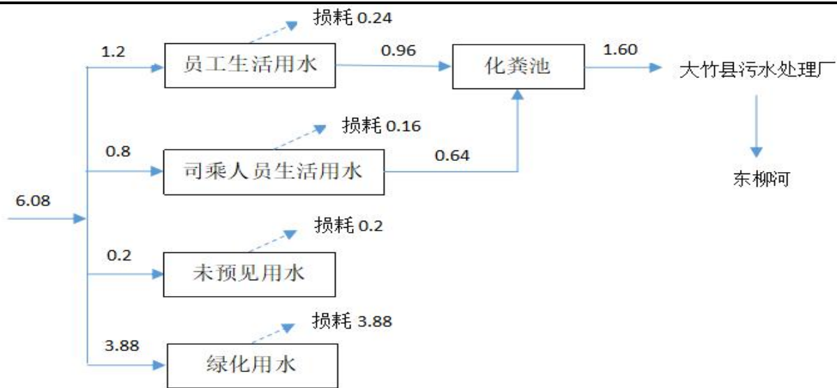
图 2-1 项目水平衡图 (消耗单位: m³/d)
