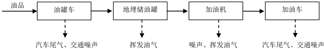
图 2-3 项目运营期产污环节框图
